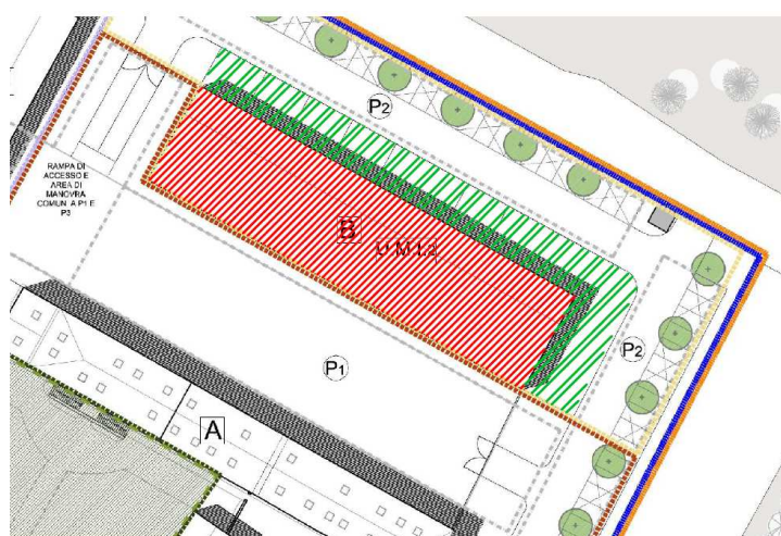
Figura 13: destinazione d'uso e relative superfici di progetto – edificio "B"
